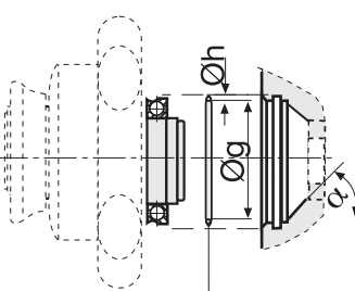
O-Ring Härte/hardness 90 shore (Lieferung auf Wunsch Delivery on request)
